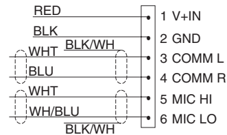
Diagramme d'interfaçage avec l'appareil
