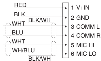
飞机接口示意图
