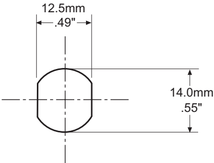
Receptáculo - Esquema de pinos (vista frontal)
